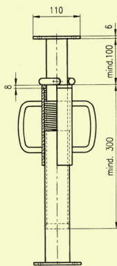
Deckenstütze A 59312 Verstellbereich 180 - 300 cm • schwere Ausführung für den harten Baustelleneinsatz • spezielles, leichtgängiges und selbstreinigendes Gewinde
