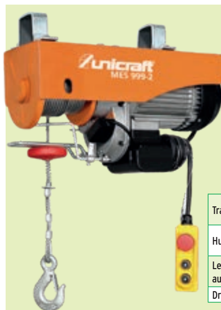
Elektro Seilzug 500/1.000 kg 48620 • inklusive Umlenkrolle • Schutzklasse IP 54
